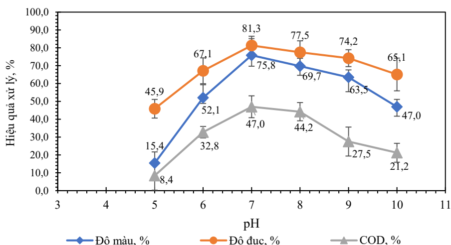
Hình 2. Ảnh hưởng của pH đến quá trình keo tụ với nồng độ phèn 45 mg/L và nồng độ COE 10 mg/L
