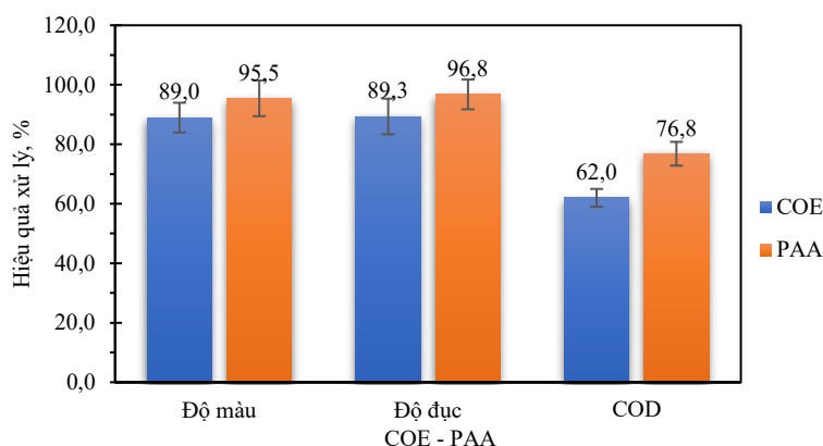
Hình 5. So sánh hiệu quả xử lý của COE và polyme thương mại PAA
