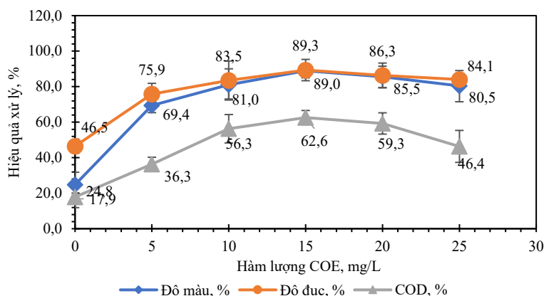
Hình 4. Ảnh hưởng của hàm lượng COE đến quá trình xử lý với nồng độ phen 75 mg/L, pH 7,0
