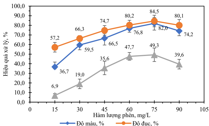
Hình 3. Ảnh hưởng của liều lượng phèn nhôm đến quá trình xử lý với nồng độ COE 10 mg/L, pH 7,0
