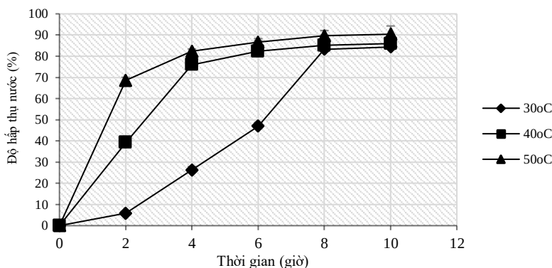
Hình 2. Ảnh hưởng của nhiệt độ và thời gian ngâm đến độ hấp thụ nước
