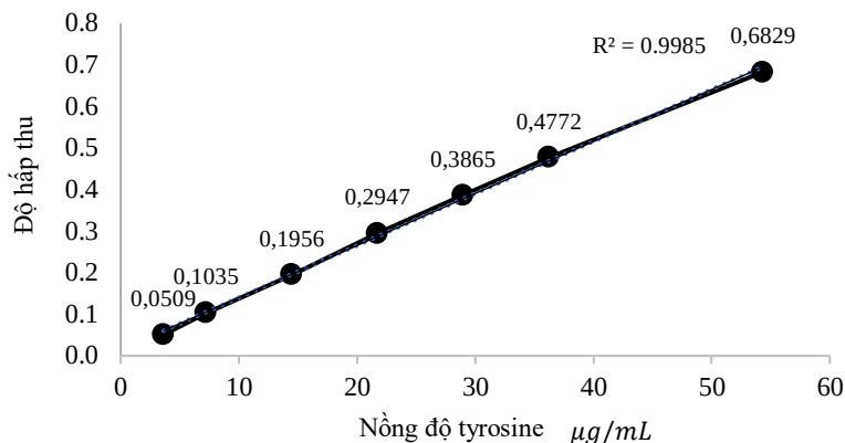
Hình 1. Phương trình đường chuẩn tyrosine
